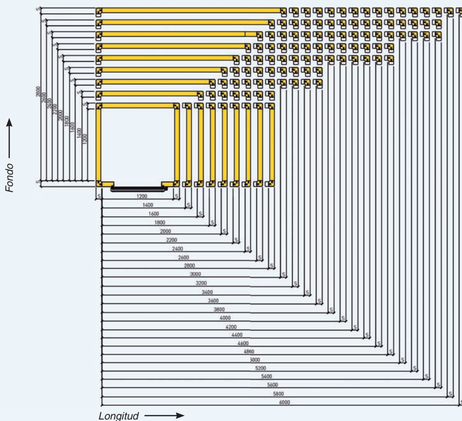
Modularidad y dimensiones Modularidad cada 200 mm
