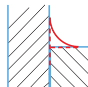
Nudo esquina sanitario y perfil radio sanitario
