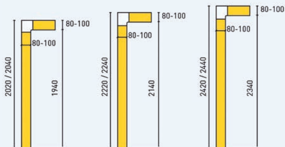
Modularidad y dimensiones Modularidad cada 200 mm
