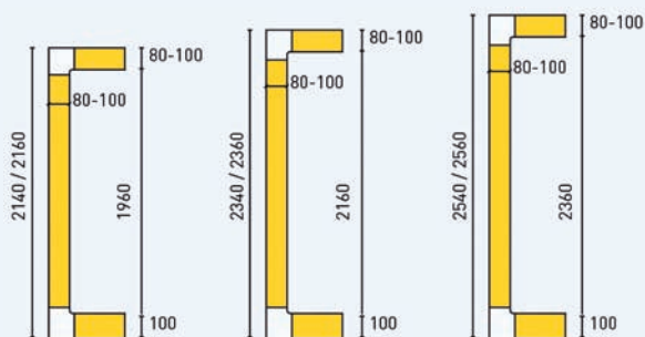
Cámaras sin suelo / Altura de cámara
